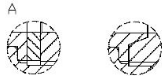
Flach dichtend Konisch dichtend
