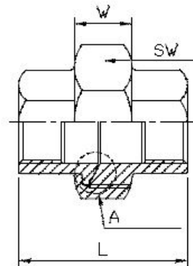
Flach dichtend Konisch dichtend
